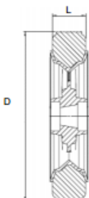
Des. 1- Dimensões do Aro de ferro 8"
