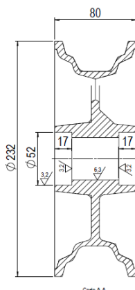
Des. 1- Dimensões do Aro de ferro 8"
