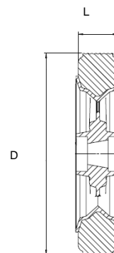
Fig.5- Estrutura e dimensões do Aro de Alumínio 4" para Rolamento
