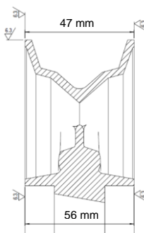
Fig.4- Ø115 mm. Estrutura e dimensões do Aro de Alumínio 4" para Rolamento sem pneu.
